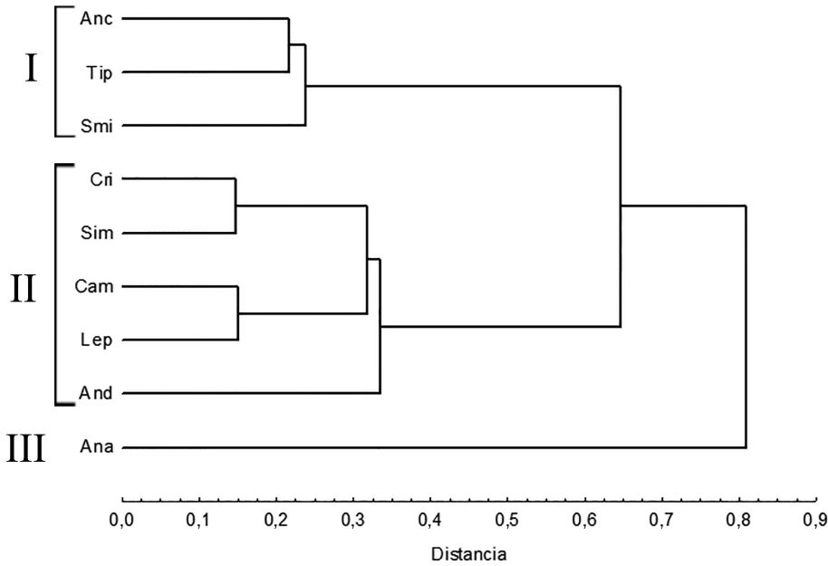
Figura 5. Análisis de conglomerados para los gremios tróficos de los nueve géneros de insectos acuáticos evaluados basado en los resultados de la composición de la dieta del ACP. Ver códigos de los géneros en la Tabla 1. I = Fragmentadores, II = Recolectores y III = Depredadores.
