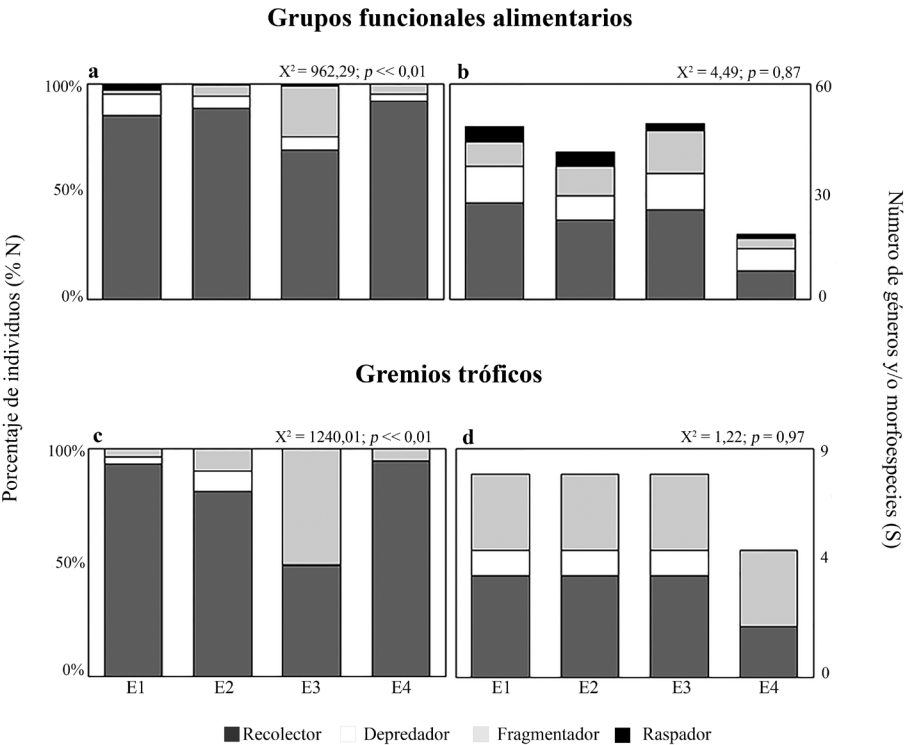
Figura 2. Grupos funcionales alimentarios (GFA) y gremios tróficos (GT) de insectos acuáticos en quebradas con impacto agrícola y minero. Se presenta el porcentaje de individuos (a y c) y número de taxones (b y d) por GFA y GT. \chi^2 = valores de la prueba chi-cuadrado para cada conjunto de datos. Ver equivalencias de los códigos de las estaciones en figura 1.
