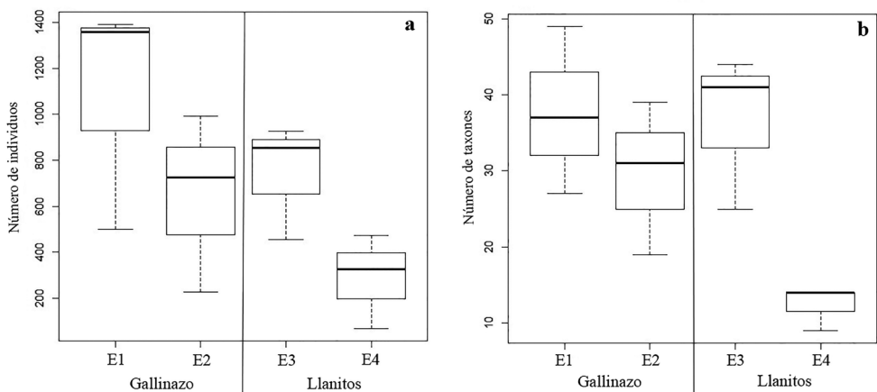
Figura 1. Gráfico de cajas y dispersión para a. abundancia y b. riqueza de insectos acuáticos entre estaciones de muestreo. E1 referencia minería, E2 minería, E3 referencia agricultura, E4 actividad agrícola.
