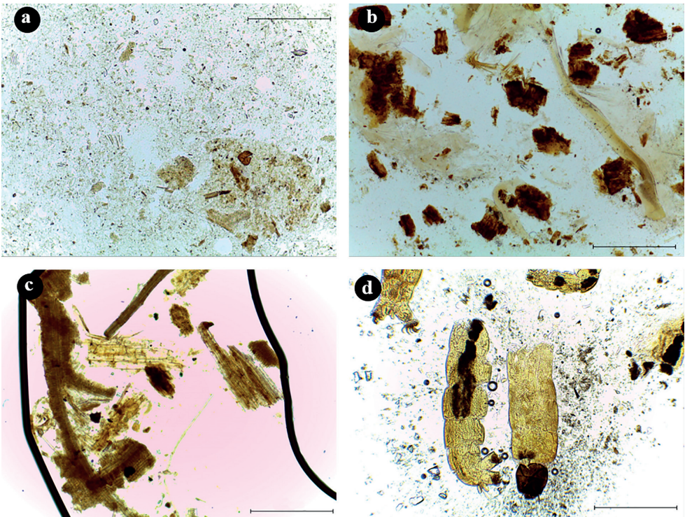
Figura 3. Principales ítems alimenticios ingeridos por los insectos acuáticos de las zonas muestreadas. a. Materia orgánica particulada fina (MOPF) en intestino de Andesiops (100x), b. Materia orgánica particulada gruesa (MOPG) en intestino de Anchytarsus (100x), c. Materia orgánica particulada gruesa (MOPG) en intestino de Tipula (100x), d. Tejido animal (T.A) en intestino de Anacroneuria (40x). Escala = 0,5mm.
